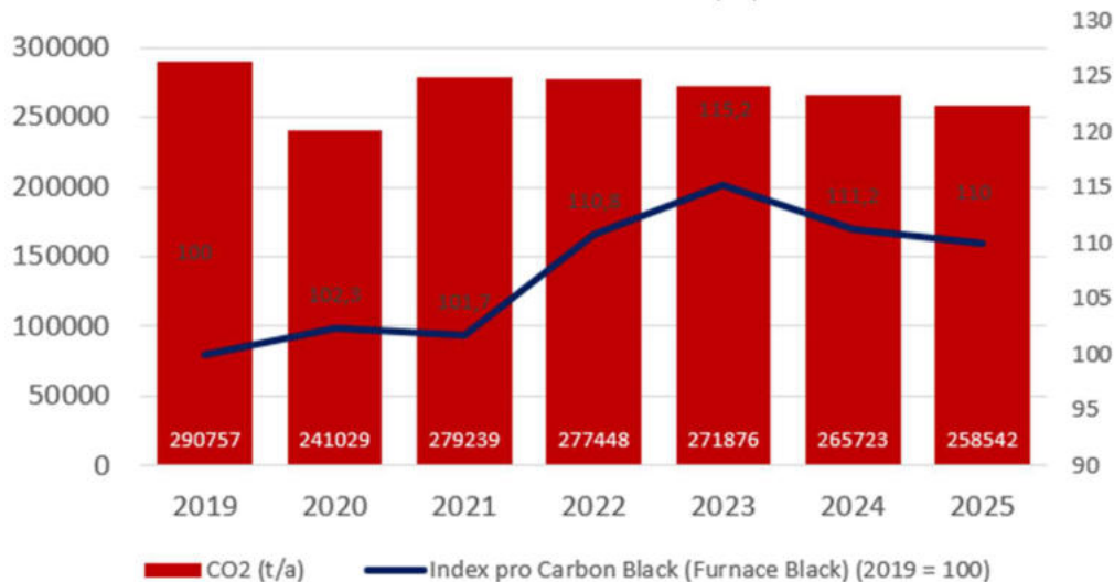
Abb. 2.19: CO 2 -Emissionen im Furnace Black-Verfahren (t/a)
