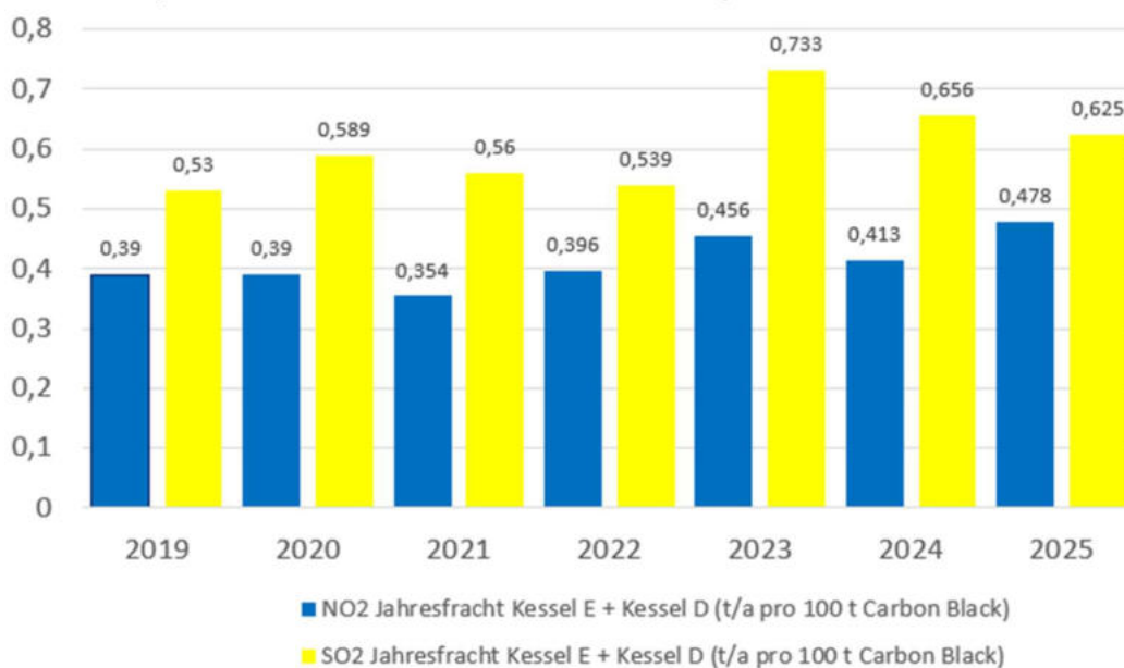
Abb. 2.20: Spezifische NO 2 - und SO 2 -Emissionen der Dampfkessel E und D
